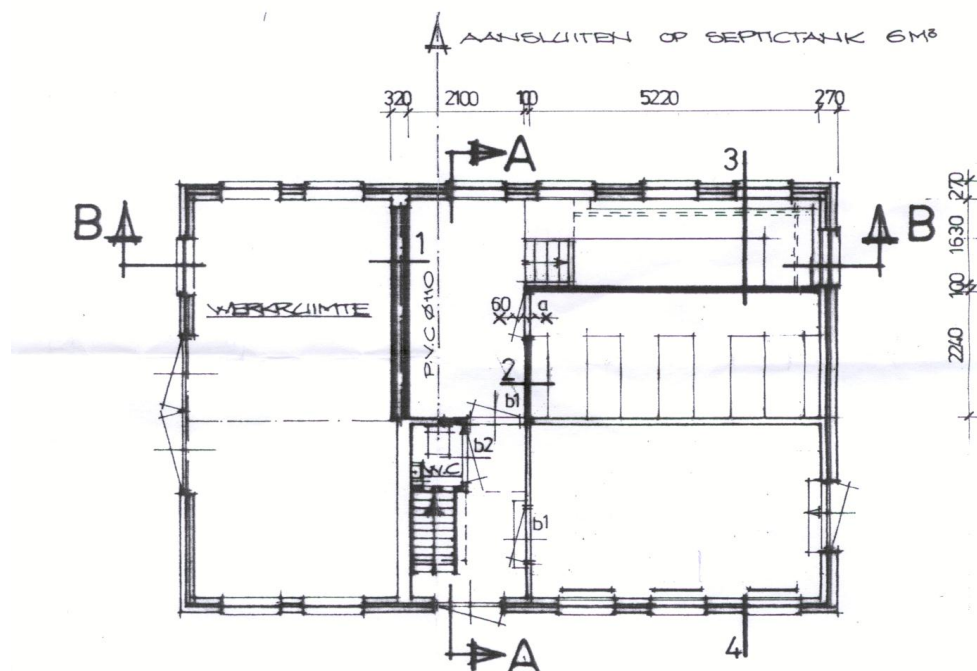
PLATTEGROND
